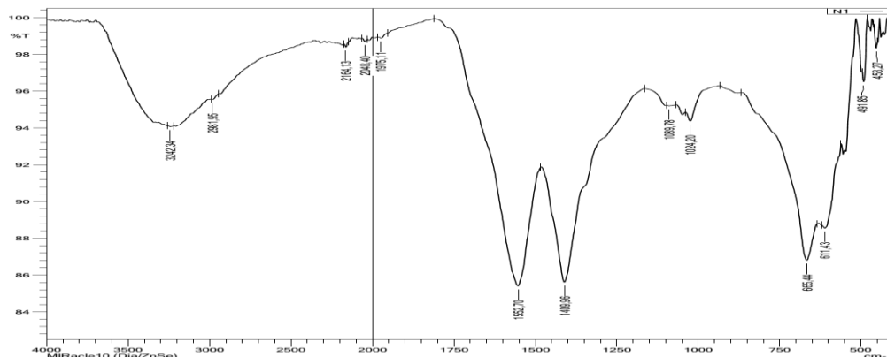
Рис.4. ИК спектр \text{NiL: NH}_3 .
