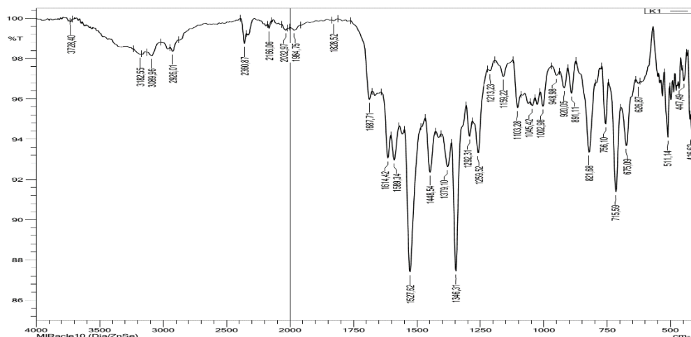
Рис.3. ИК спектр \text{CuL: NH}_3 .
