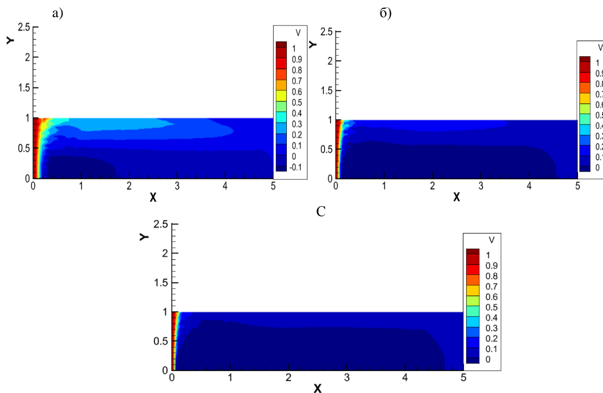
Рисунок 5. Профиль продольной скорости при большом степени закрутки
